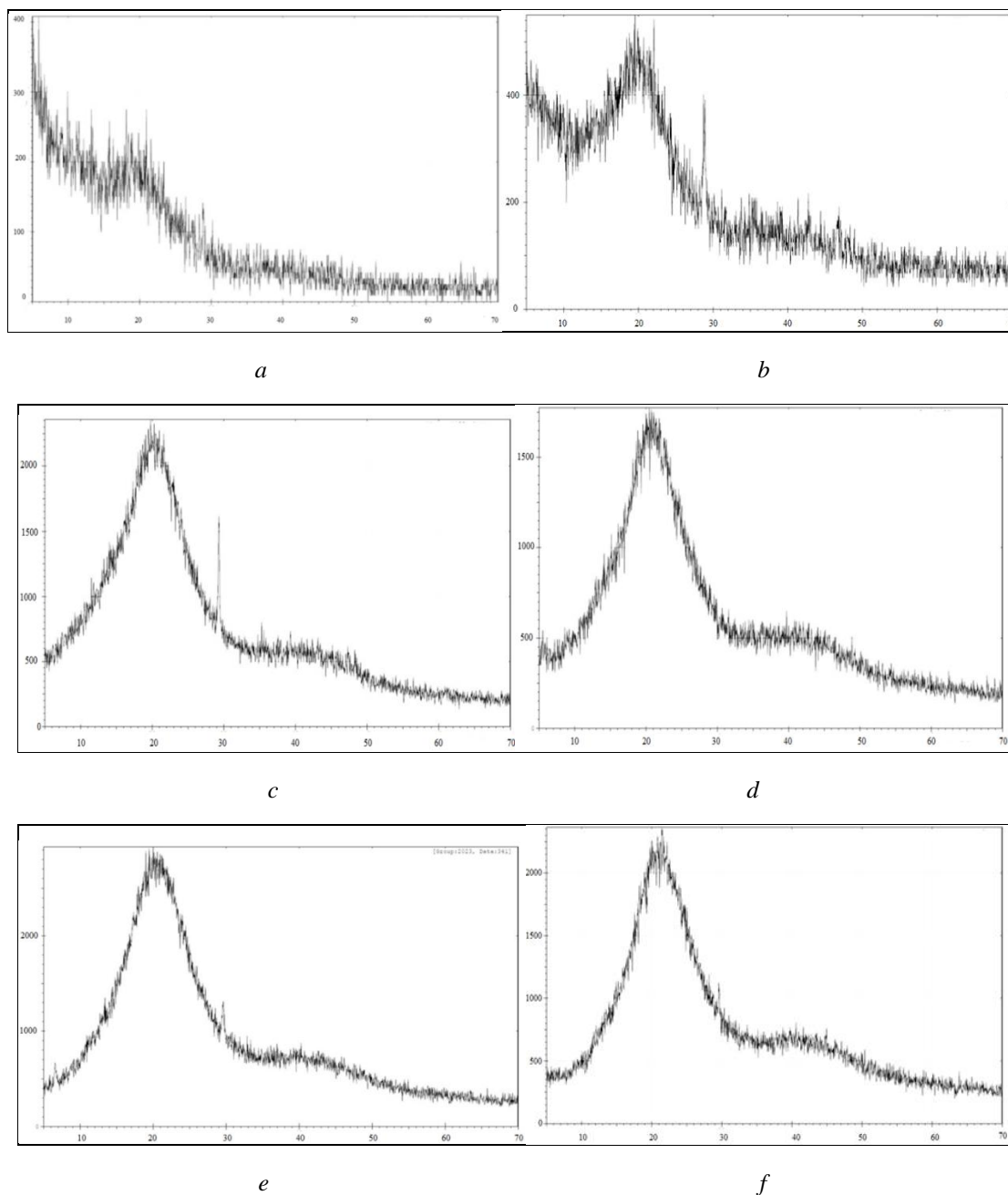
Fig. 1. X-Ray Diffraction patterns of (a) pure blend, (b) blend + ZnO NPs (1 wt. %), (c) blend + nZnO (1.5 wt. %), (d) blend + ZnO NPs (2 wt. %), (e) blend + ZnO NPs (2.5 wt. %), and (f) blend + ZnO NPs (3 wt. %)
